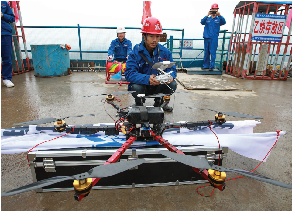
当日，由中铁广州局承建的贵州瓮（瓮安）开（开阳）高速公路开州湖特大桥先导索由无人机牵引成功，标志着大桥即将进入桥梁主缆架设阶段。 据了解，目前国内悬索桥先导索牵引通常采用火箭抛送、船舶拽拉、热气球牵引和直升机牵引等施工方法。结合山区峡谷的建设实际，开州湖特大桥东、西主塔“牵手”选择了无人机牵引先导索方案。 新华社记者刘续摄
